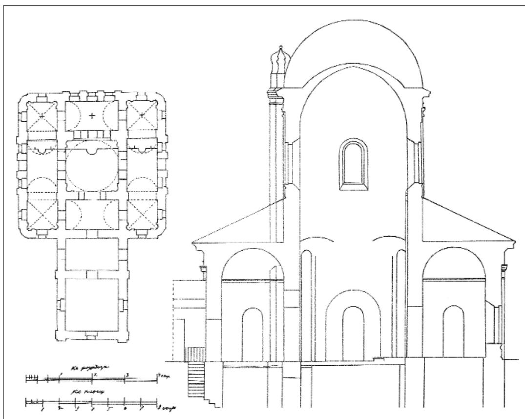
План и разрез Богородицерождественской церкви в селе Надовражино. 1905 год. Чертеж из фондов ЦИАМ
