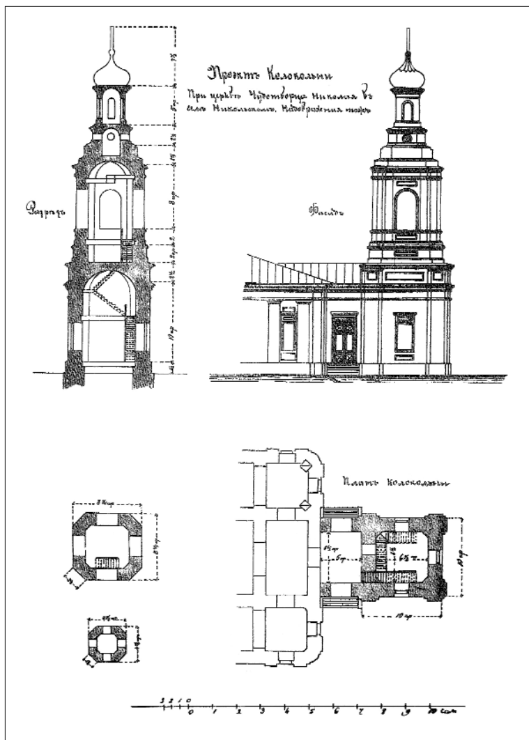
Проект колокольни церкви в селе Надовражино. 1884 год. Чертеж из фондов ЦИАМ
