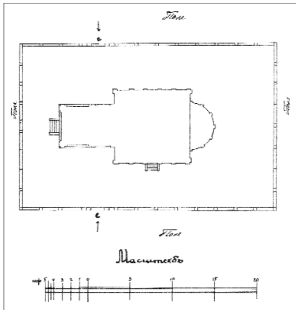
План Богородицкой церкви. 1901 год. Чертеж из фондов ЦИАМ
