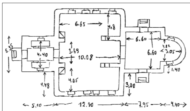
План каменной Крестовоздвиженской церкви. 1933 год. Чертеж из фондов ЦГАМО
