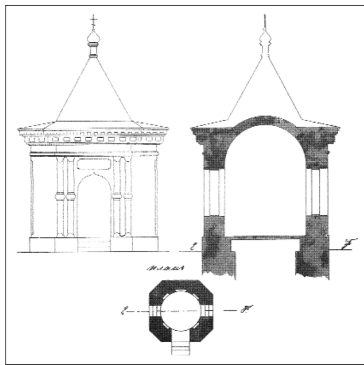
Часовня в деревне Покровское. Чертеж из фондов ЦИАМ
