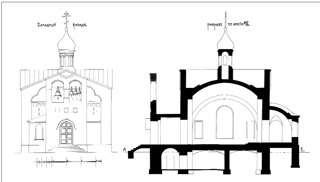
Проект нестроенного каменного храма. 1912 год. Чертеж из фондов ЦИАМ
