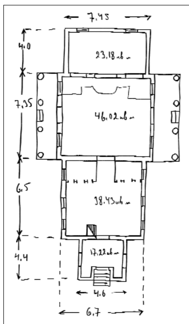
План деревянной Троицкой церкви 1931 год. Чертеж из фондов ЦГАМО
