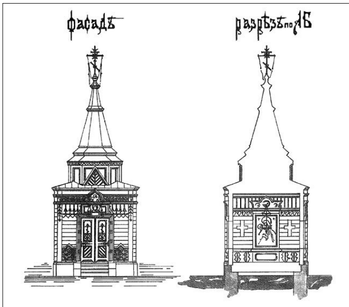
Чертеж деревянной часовни в деревне Борисово. Из фондов ЦИАМ
