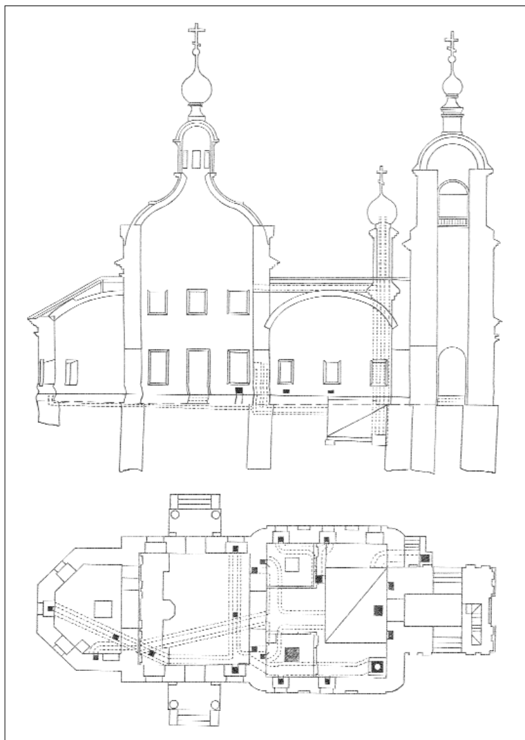
Проект духового отопления церкви в селе Савельево. 1905 год. Чертеж из фондов ЦИАМ
