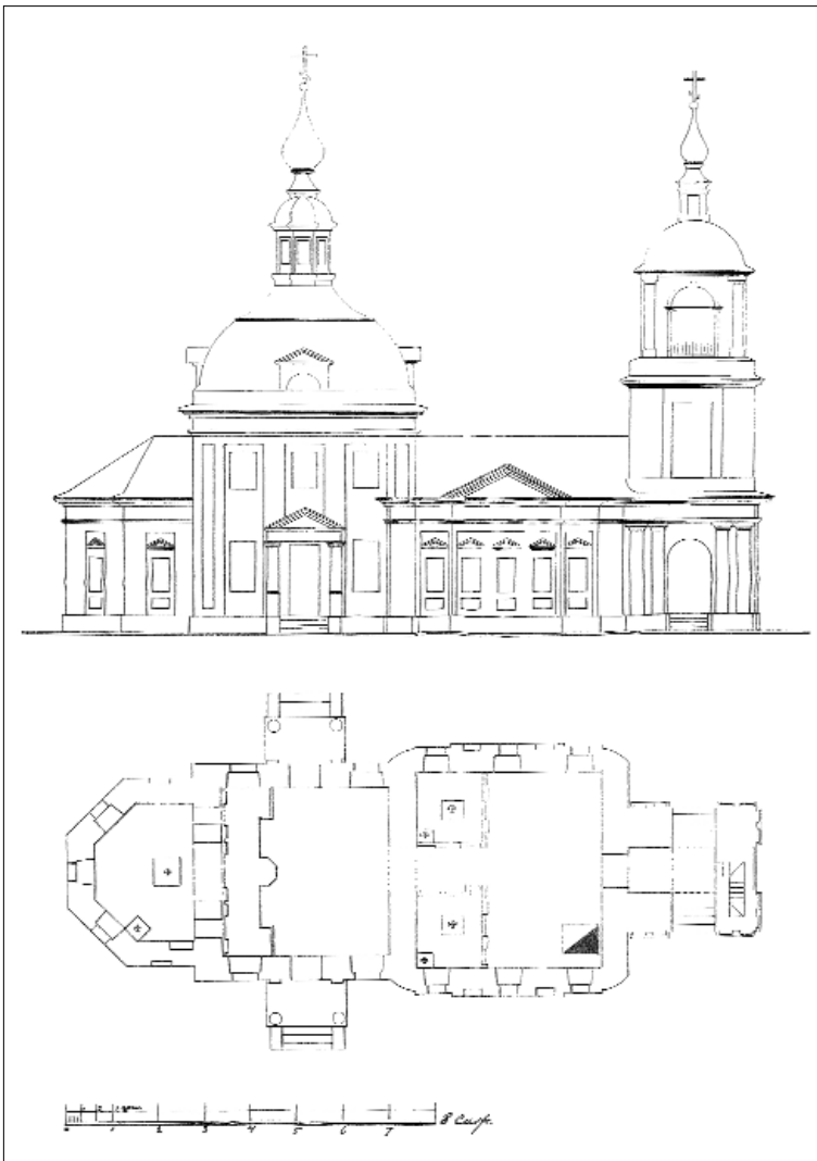
Северный фасад и план церкви в селе Савельево. 1901 год. Чертеж из фондов ЦИАМ
