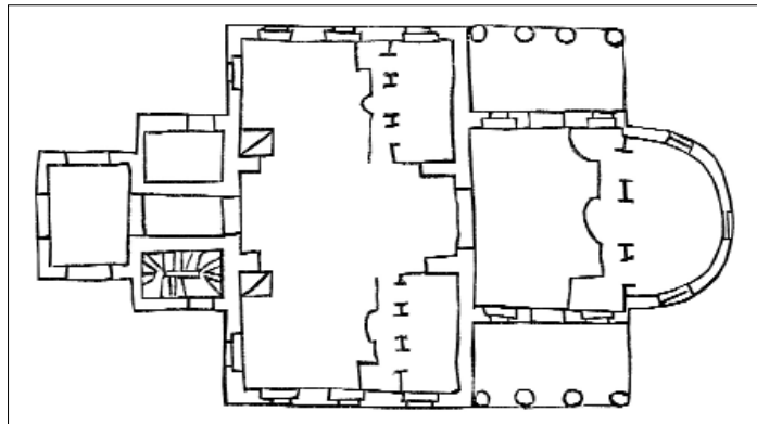
План каменной Богородицерожественской церкви. 1933 год. Чертеж из фондов ЦГАМО
